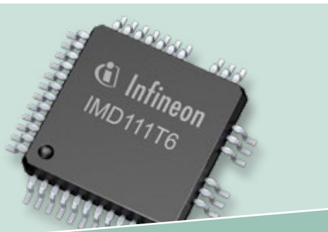
Der iMOTION™ IMD11T6 ist ein hochintegrierter IC zur Steuerung von dreiphasigen, bürstenlosen Gleichstrommotoren.
